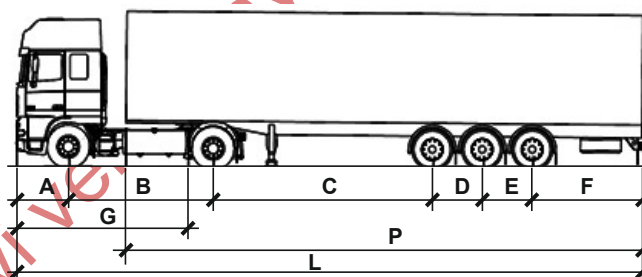
F77. ábra – Mértékadó nyerges járműszerelvénny méretei
