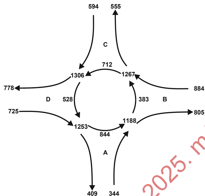
F66. ábra – Vonalas forgalomáramlási ábra
