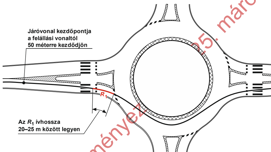
13. ábra – A járóvonal körforgalomba történő belépési sugarának mérése
