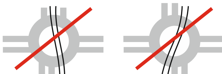
38. ábra – Körpályát keresztező villamosvágány tiltott kialakítása
