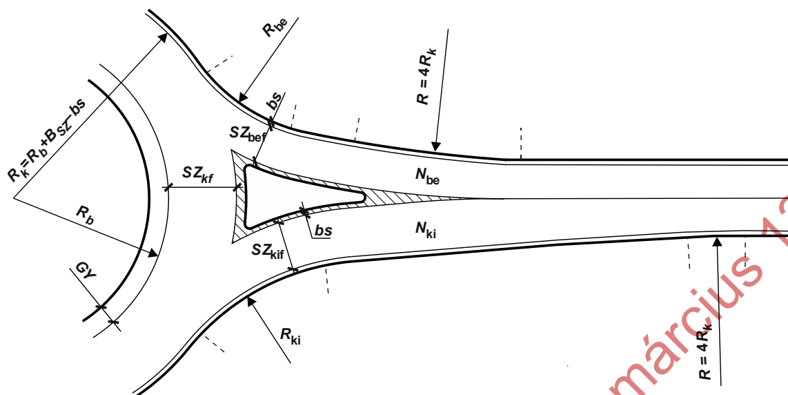
44. ábra – Csomóponti ág típusrajza
