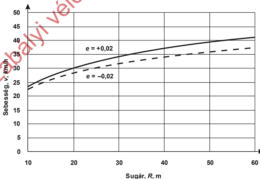
F59. ábra – Sebesség és ívsugarak kapcsolata
