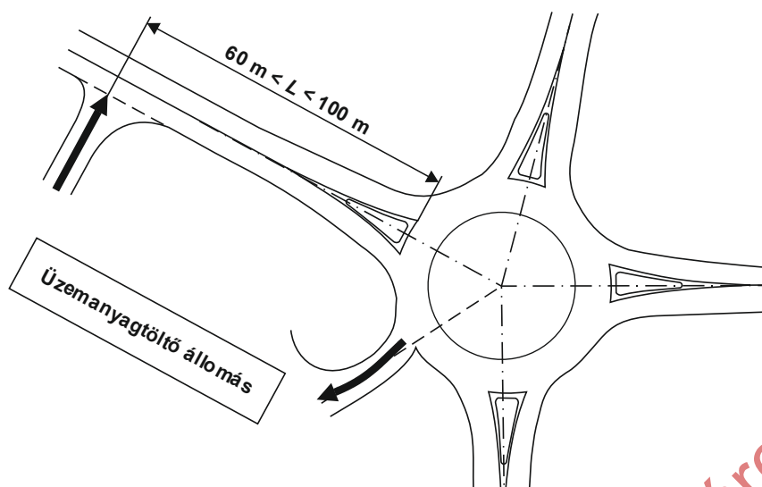
35. ábra – Közúti üzemmel kapcsolatos létesítmények csatlakoztatása III.
