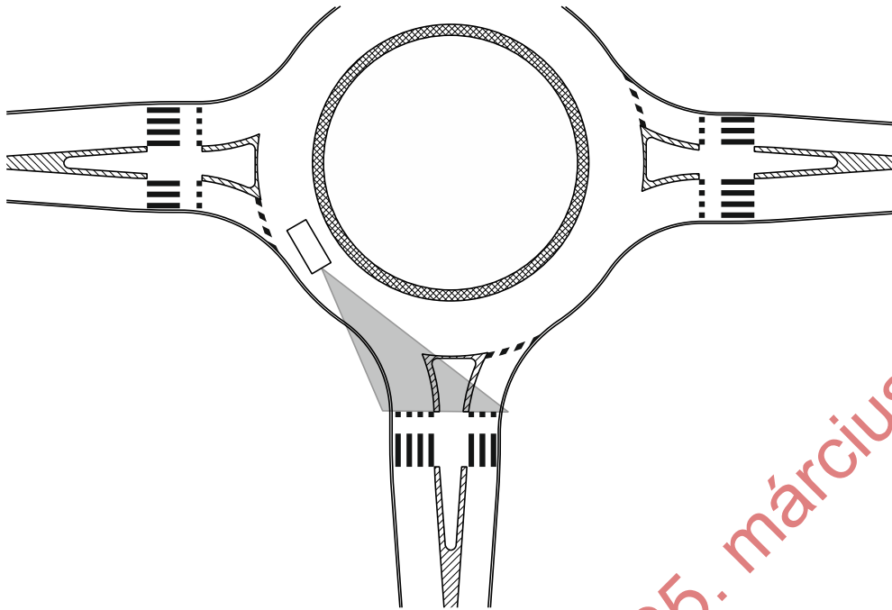
16. ábra – Látómező és szabadon tartandó tér a körpályán haladó jármű szempontjából kijelölt gyalogos-átkelőhely esetén
