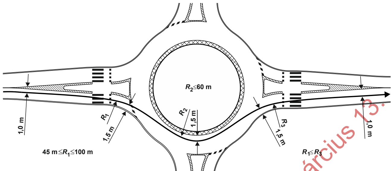
11. ábra – Kitérítés egysávos körforgalomnál egyenes áthaladás esetén
