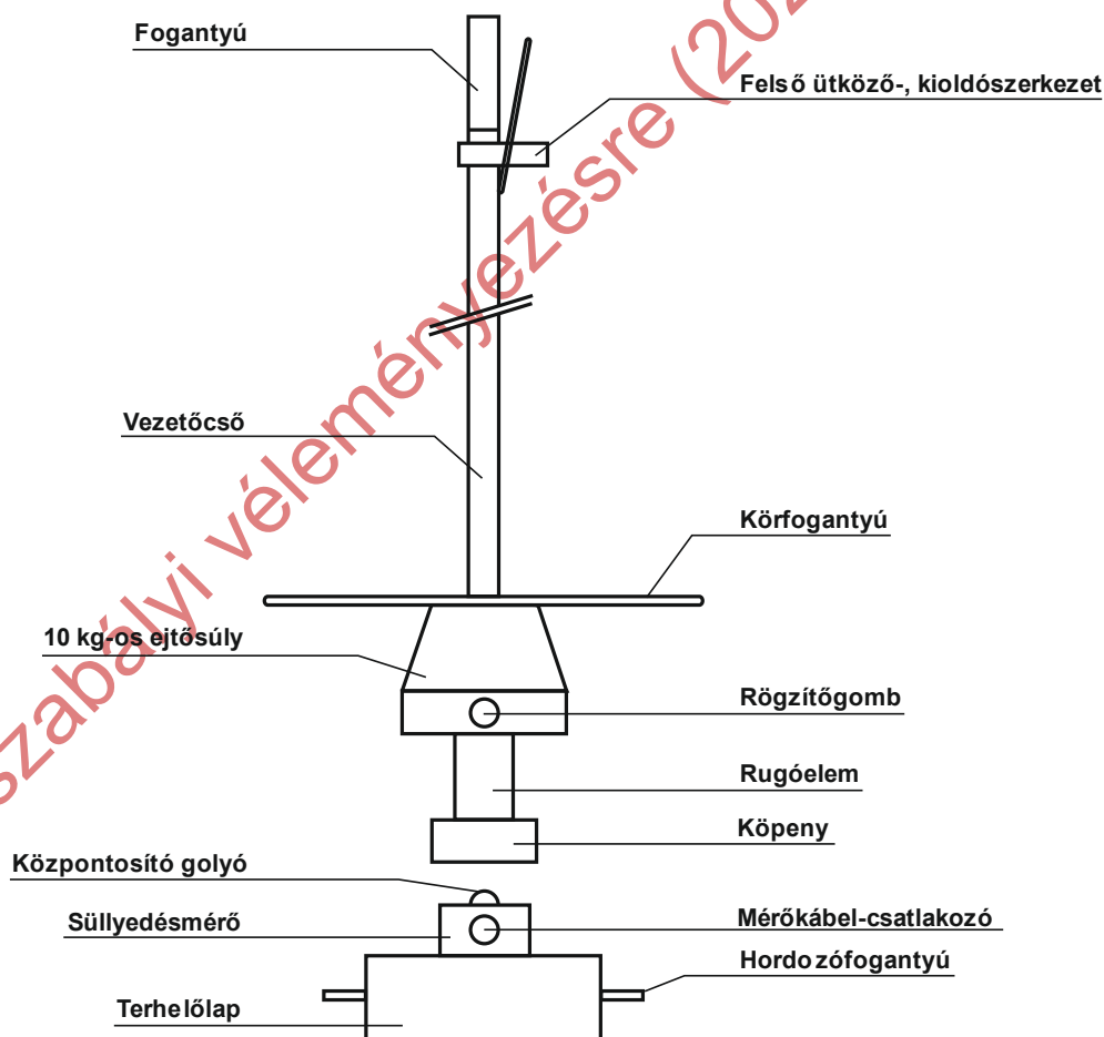
2. ábra – Könnyű ejtősúlyos mérőberendezés elvi rajza
